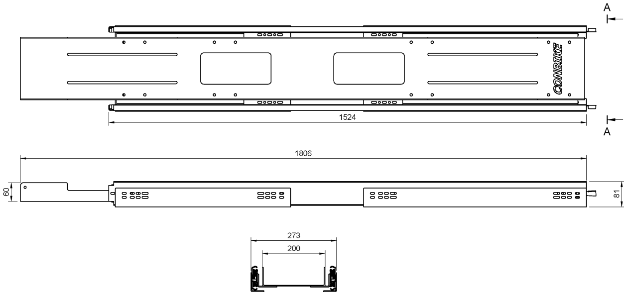
A-A
